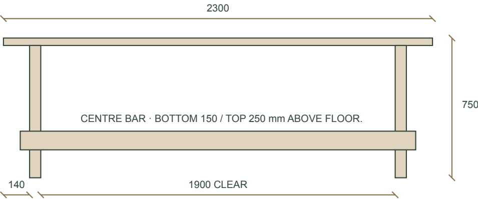
03 / LONG SIDE
